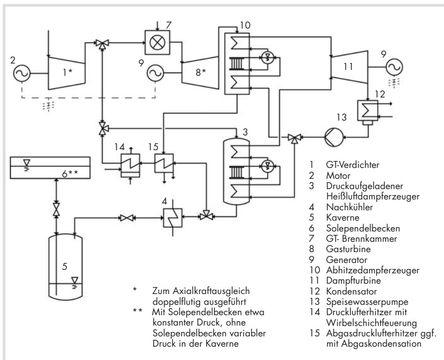
Bild 8. Isobares GuD-Druckluftspeicherkraftwerk mit direkter Umwandlung der Kompressionswärme [Leithner 2011].
