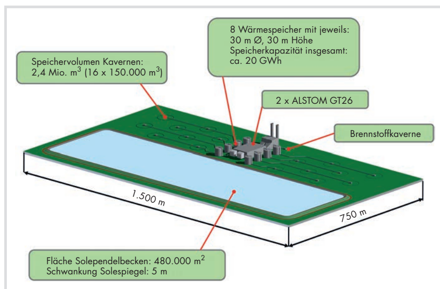
Bild 4. Beispielhafter Aufstellungsplan im Gelände [Nielsen, Leithner 2012].
