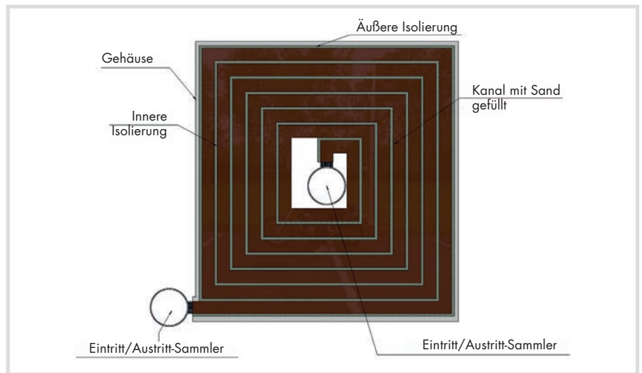
Bild 5. Spiralförmiger Schichtwärmespeicher [Qi 2013].
