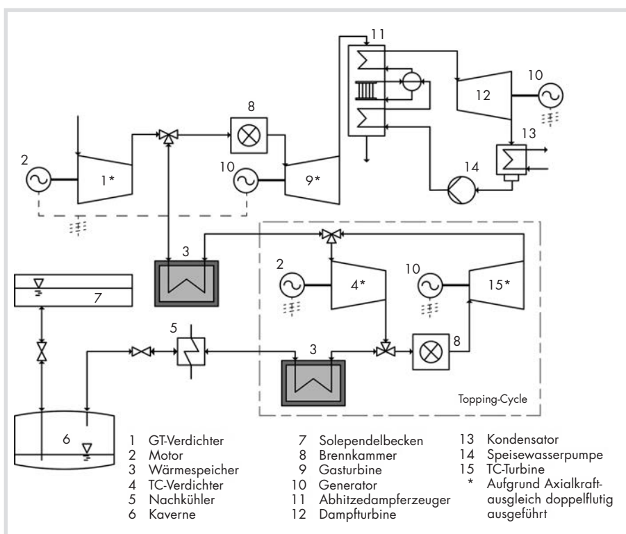
Bild 7. Teilisobares GuD Druckluftspeicherkraftwerk mit Topping-Cycle und 2 Wärmespeichern [Leithner 2007], [Nielsen 2013].
