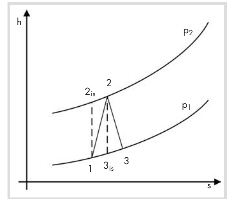
Bild 2. Polytrpe und isentrope Kompressionen und Expansionen [Leithner et al. 2014].
