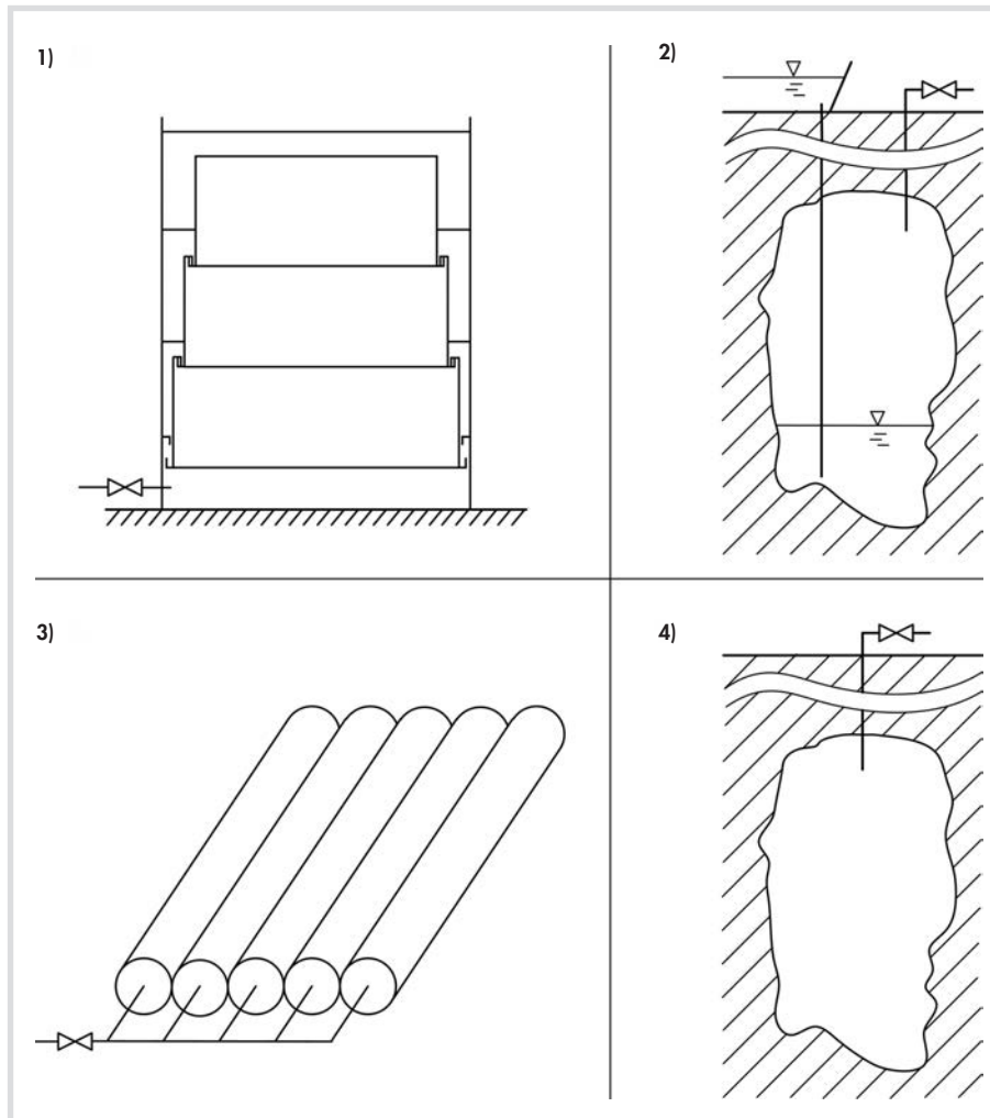
Bild 1. Isobare Speichervolumina (1: Gasometer, 2: Salzkaue mit Solependelbecken) und isochore Speichervolumina (3: Pipelineröhren, 4: Salzkaue) [Leithner et al. 2014].
