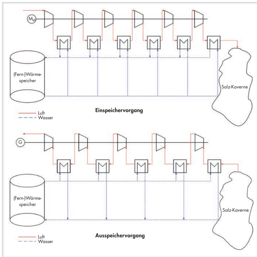
Bild 9. Druckluftspeicherkraftwerk mit Niedertemperaturwärmespeicher ohne Dampfkreislauf [Oldhafer et al. 2014].
