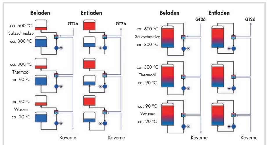
Bild 6. 6-Tank und 3-Tank Thermocline Wärmespeicher bzw. 4-Tank und 2-Tank Thermocline Wärmespeicher ohne Wasser (vorausgesetzt das Thermoöl ist bei 20 °C ausreichend dünnflüssig, sodass es umgepumpt werden kann [Nielsen et al. 2011]).
