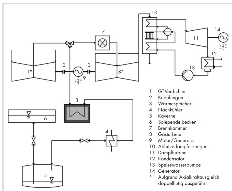
Bild 3. Isobares GuD Druckluftspeicherkraftwerk mit Wärmespeicher, ISACOAST-CC [Isobaric Adiabatic COmpressed Air Energy Storage – Combined Cycle] Prinzipskizze [Leithner 2006], [Nielsen 2013].
